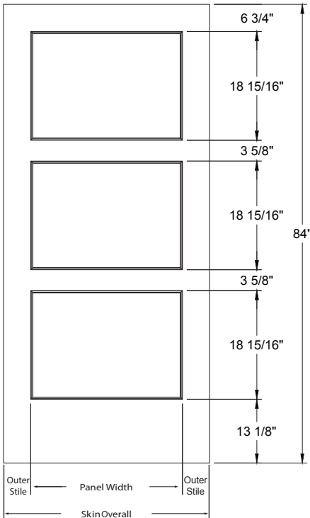
DOOR SKIIN DIMENSIONS*
